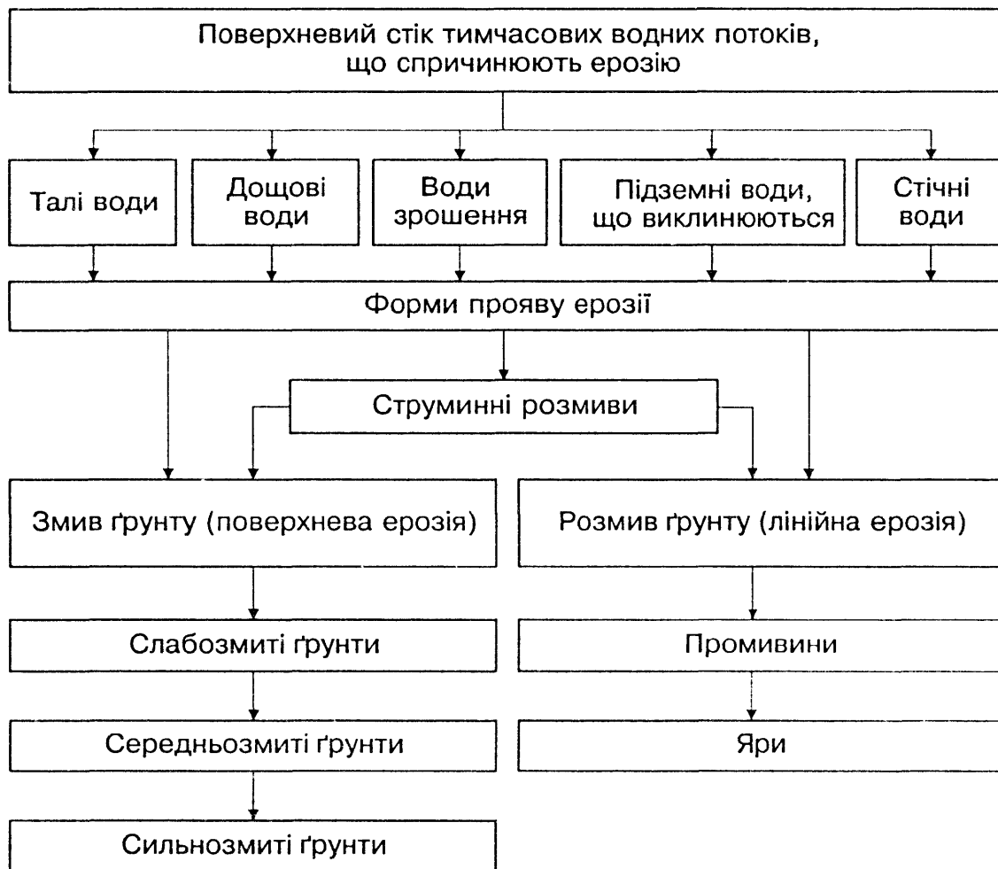
Рис. 8.3 - Класифікація ерозії ґрунтів (за М. М. Заславським)
