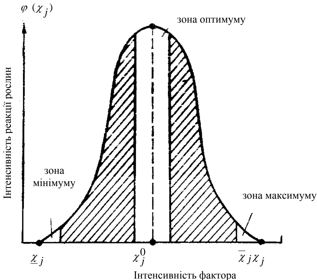
Рис. 4.6 – Схема дії температури повітря на рослини (за К.М.Ситником, А.В.Брайоном, О.В.Городецьким). x_j – точка мінімуму, x_j^0 – точка оптимуму; \bar{x}_j – точка максимуму.
