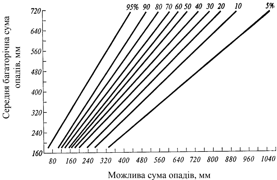
Рисунок 10.5 – Графік для розрахунку сум опадів різної забезпеченості за рік (за А.М. Лебедєвим)
