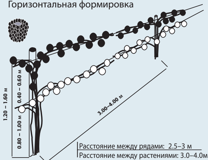
Горизонтальная формировка
